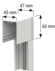
Rail haut
