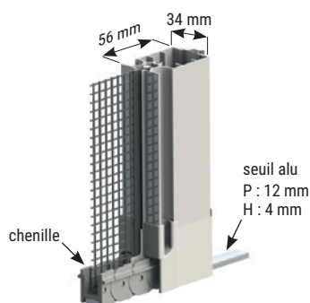
Coffre
